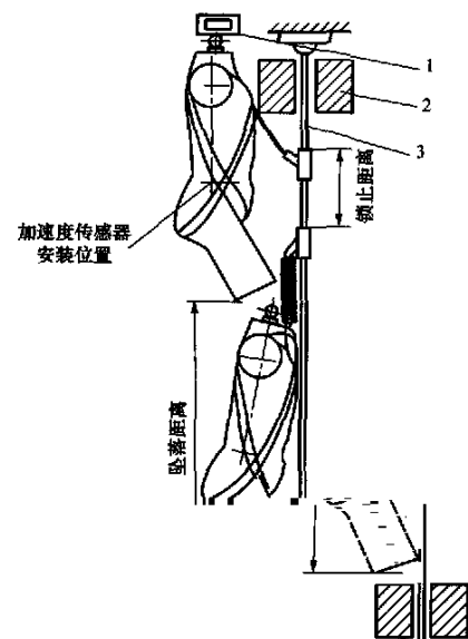
图 A.1 速差式防坠器试验布置图
