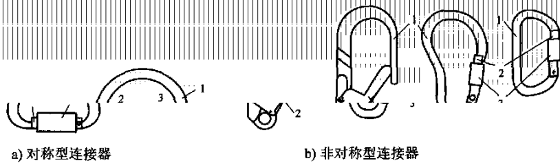
图 3 连接器结构示意图
